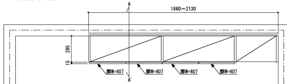
平面図（上部）
