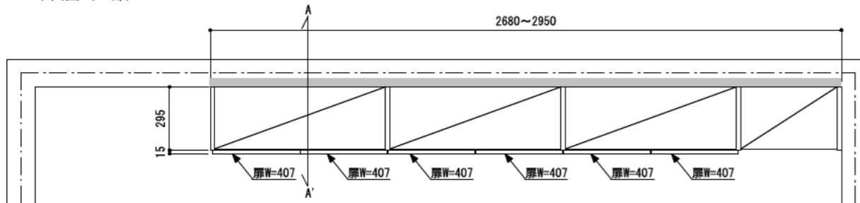
平面図（上部）
