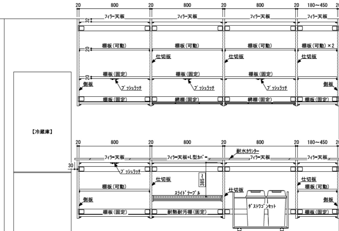
正面図（扉内部）
