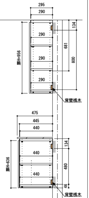
A-A' 断面
