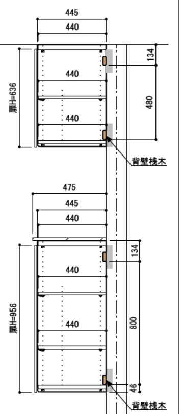
A-A' 断面
