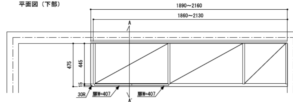
平面図（下部）
