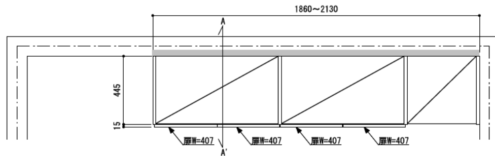
平面図（上部）
