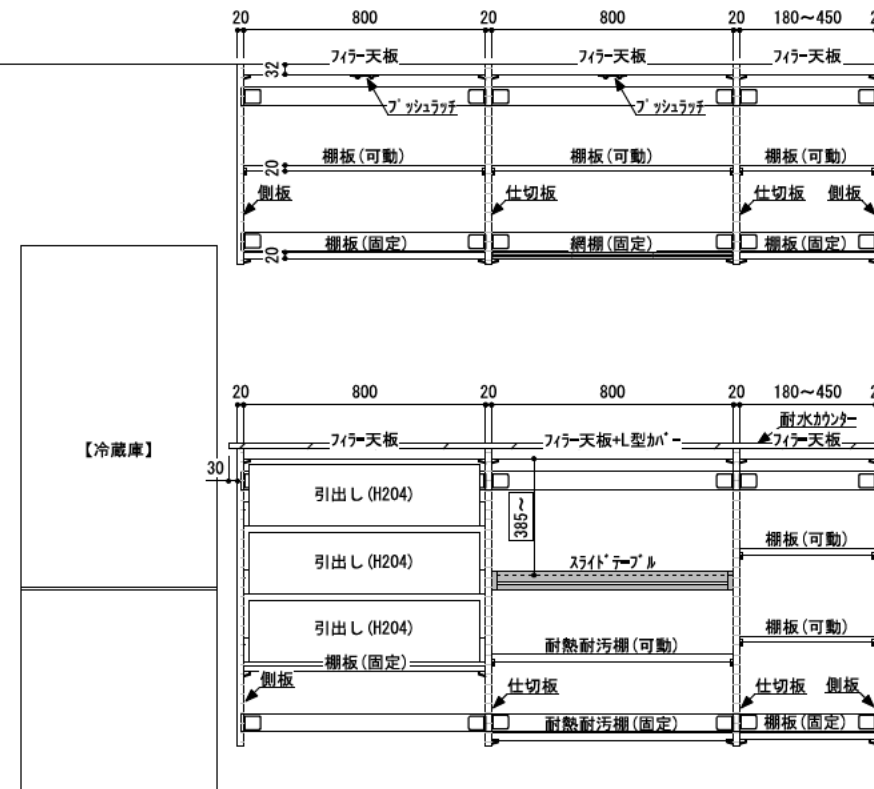
正面図（扉内部）
