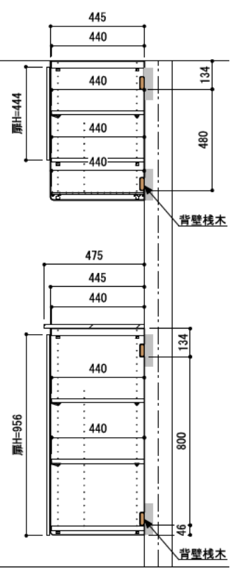
A-A' 断面
