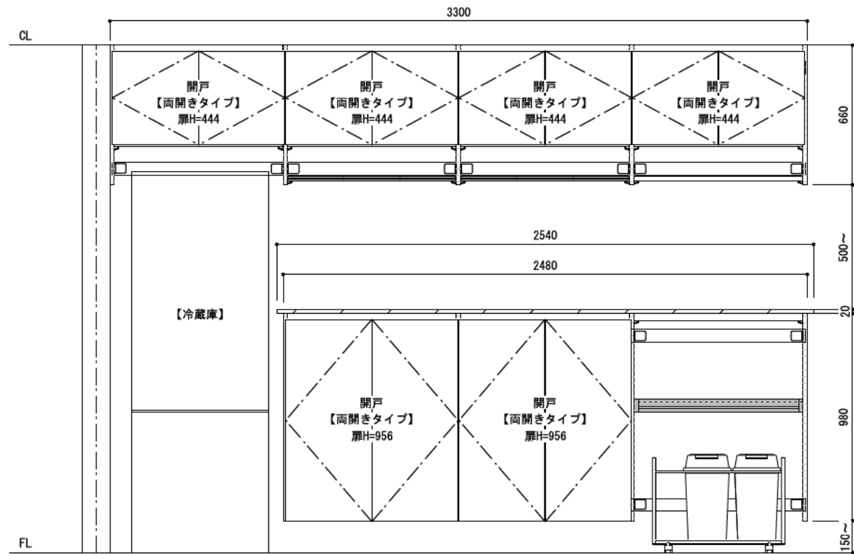
正面図（外観）
