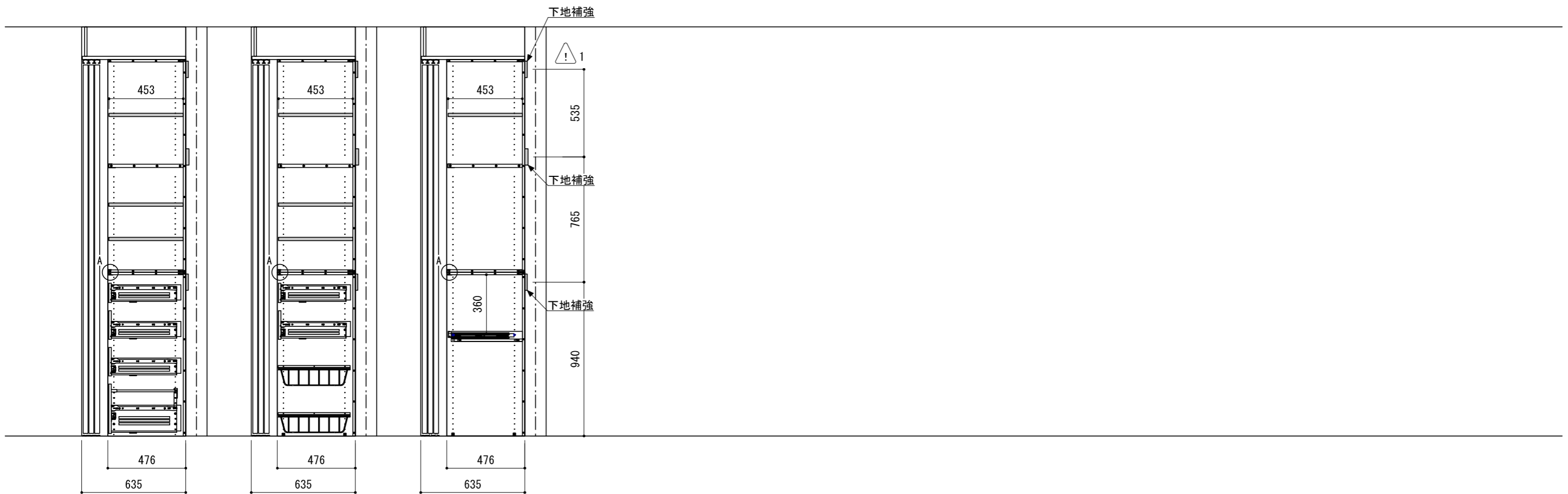
A-A' 断面
