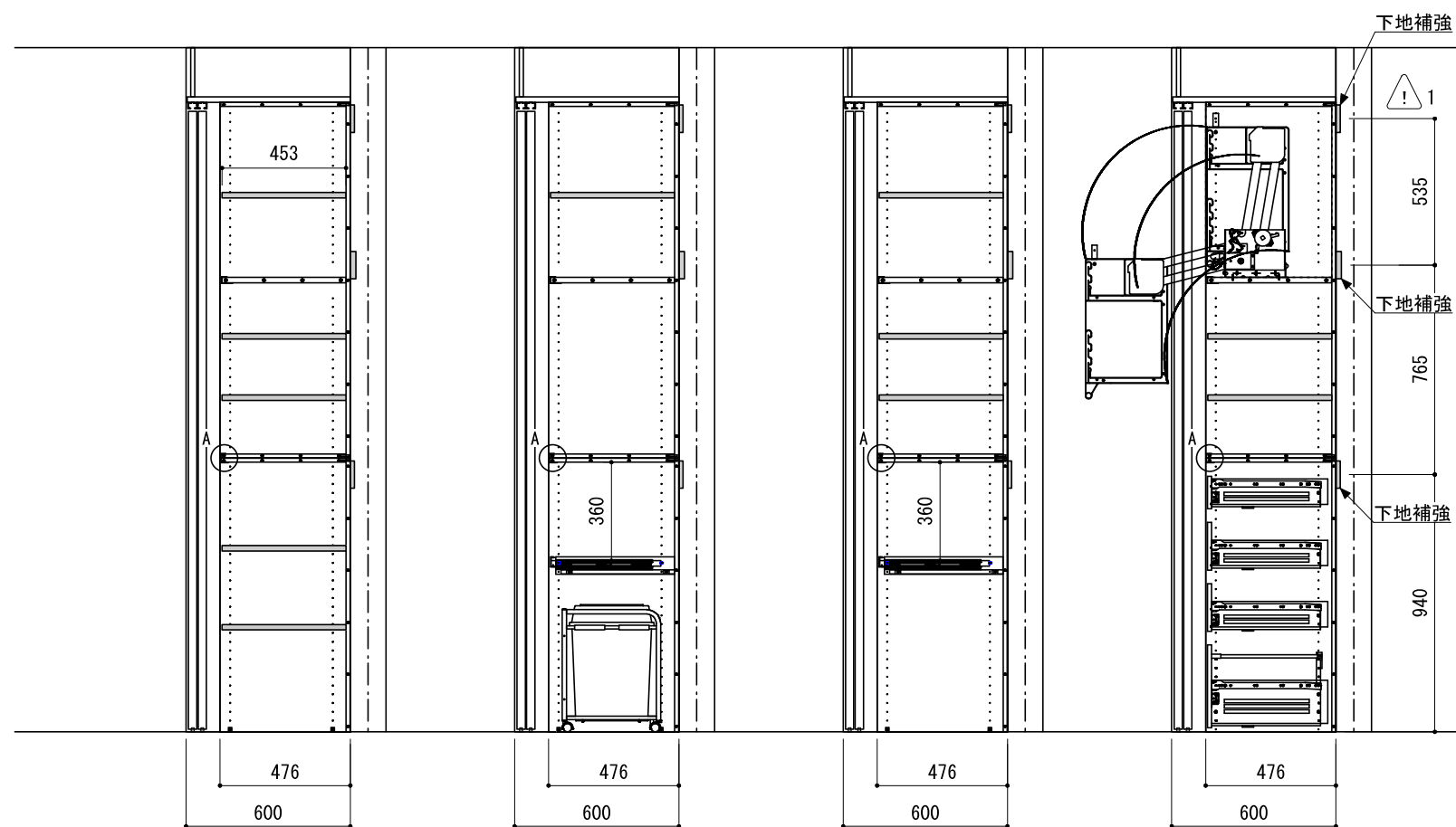
A-A' 断面
