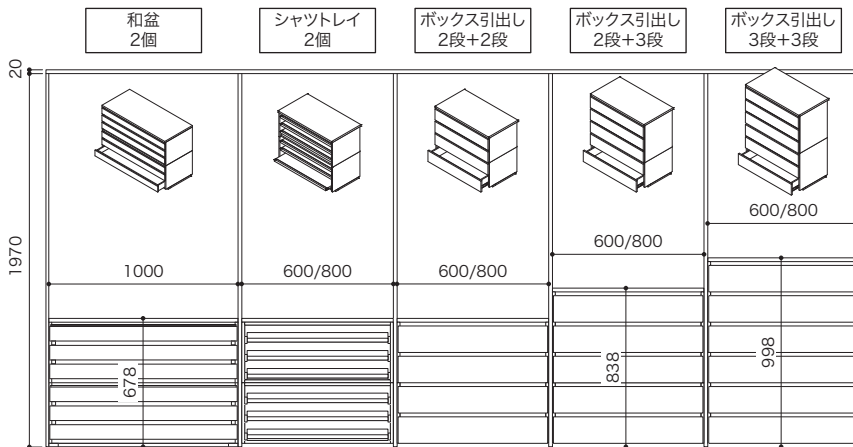
[正面図]
